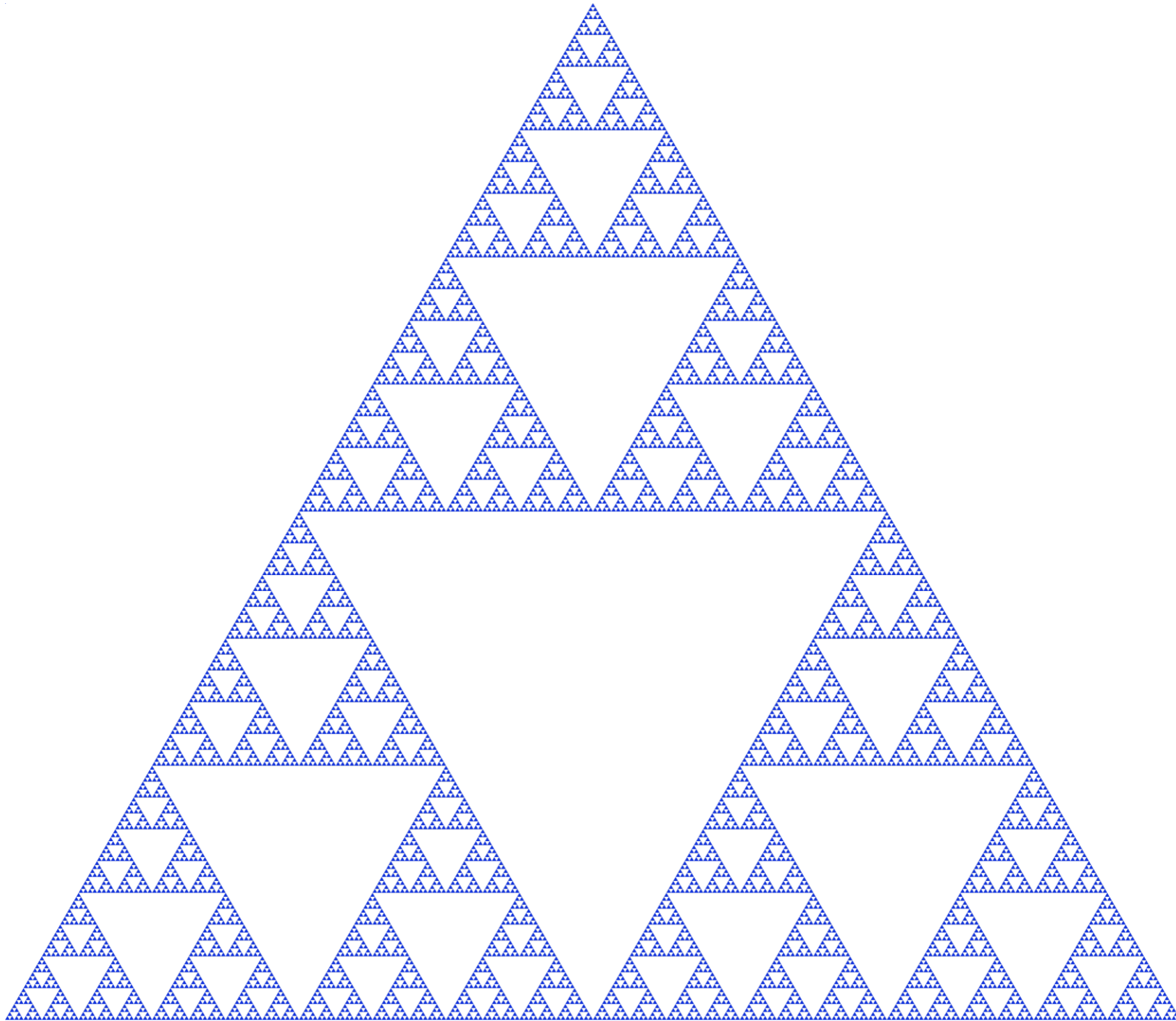
Sierpinski triangle
